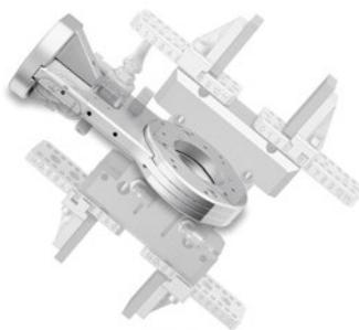
D180: Dual Gripper 180°
